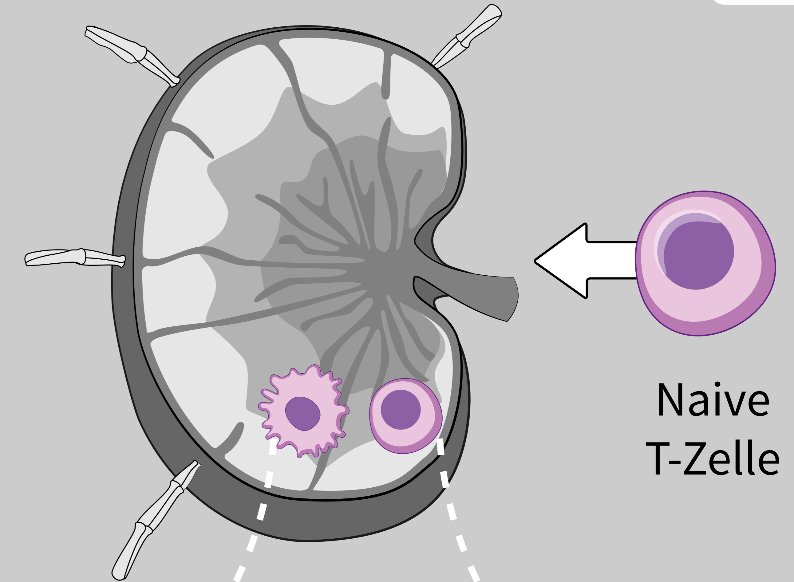
Lymphknoten
