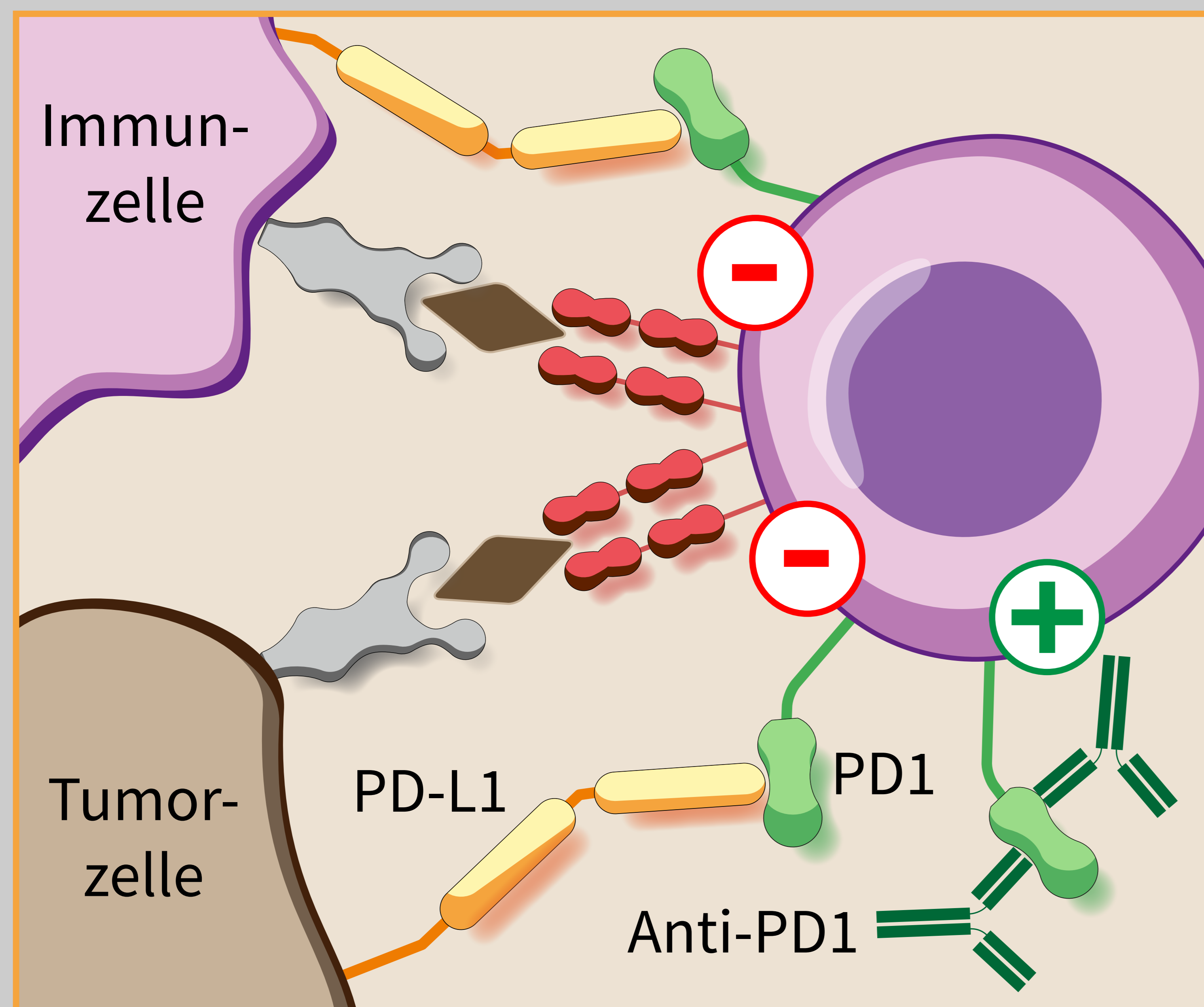
Tumormikroumgebung
